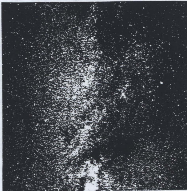
Stjärnmoln i Vintergatans
